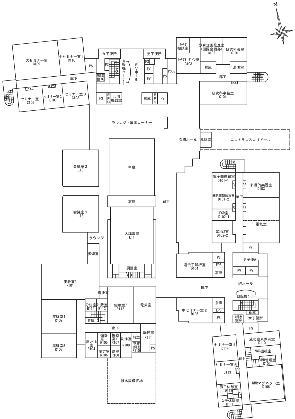
1 F 平面図
